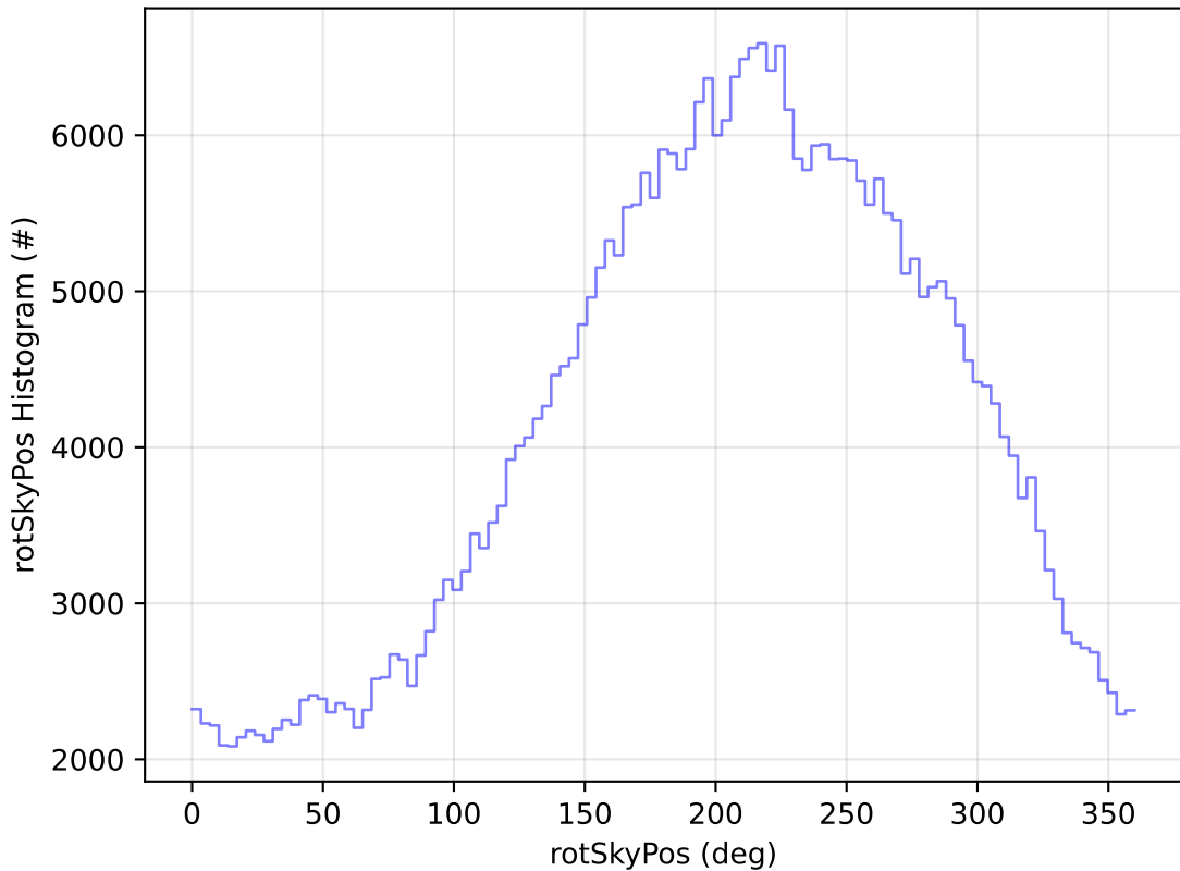
too_elab_r256_d2_ugrizy_v3.4_10yrs WFD z band: rotSkyPos Histogram
