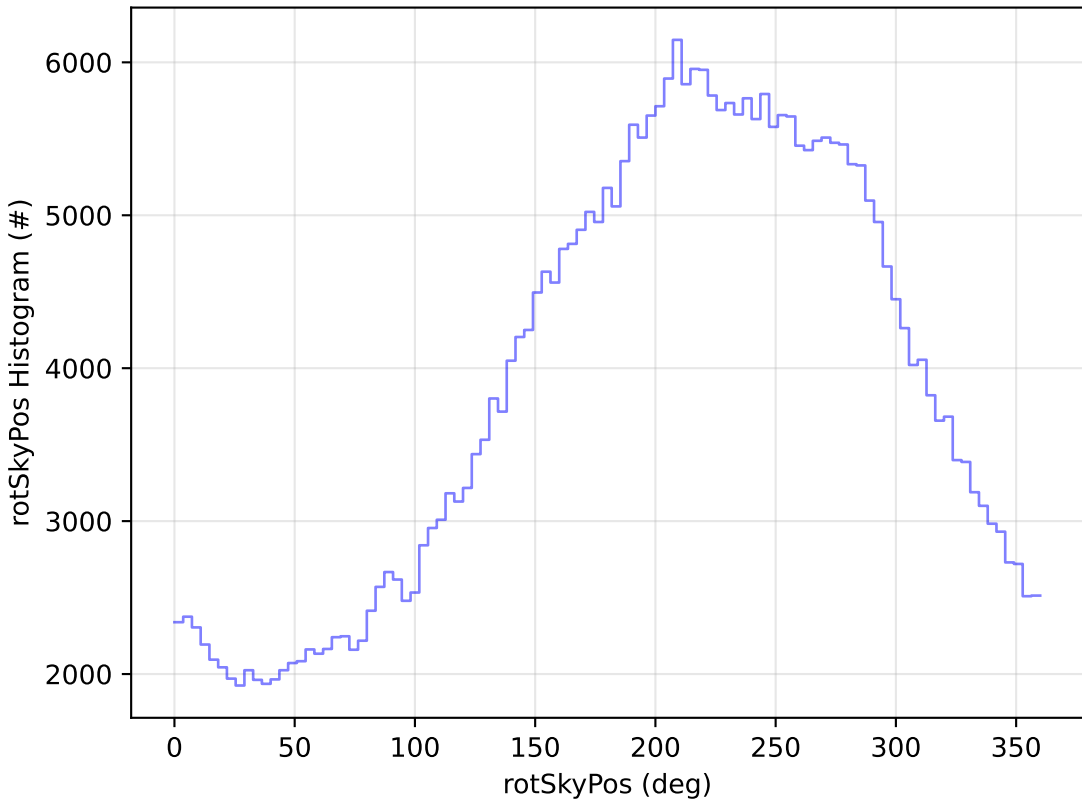
too_elab_r256_d2_ugrizy_v3.4_10yrs WFD y band: rotSkyPos Histogram
