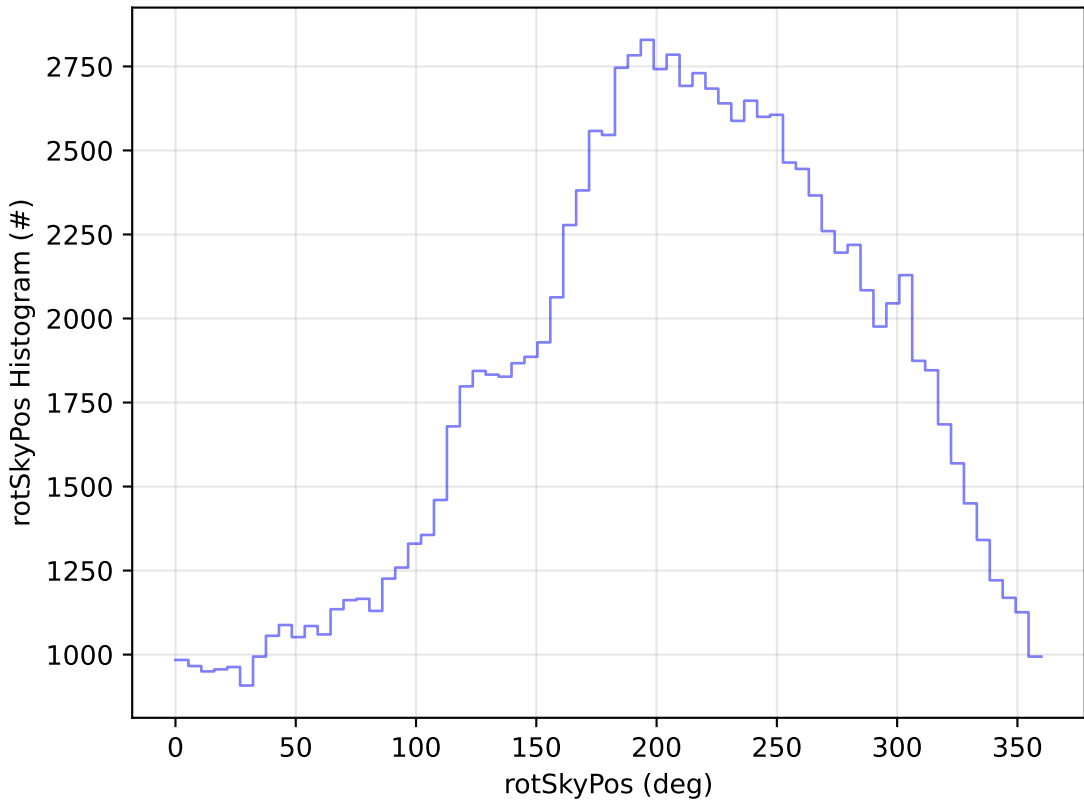
too_elab_r256_d2_ugrizy_v3.4_10yrs WFD u band: rotSkyPos Histogram
