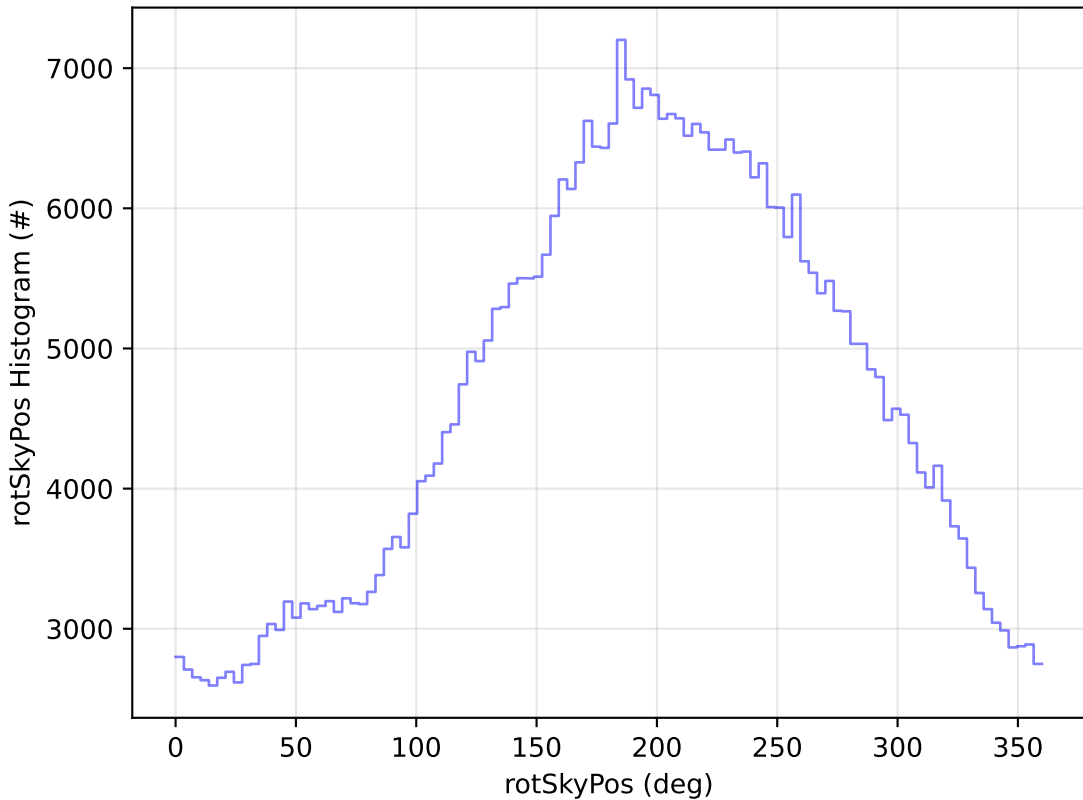
too_elab_r256_d2_ugrizy_v3.4_10yrs WFD r band: rotSkyPos Histogram
