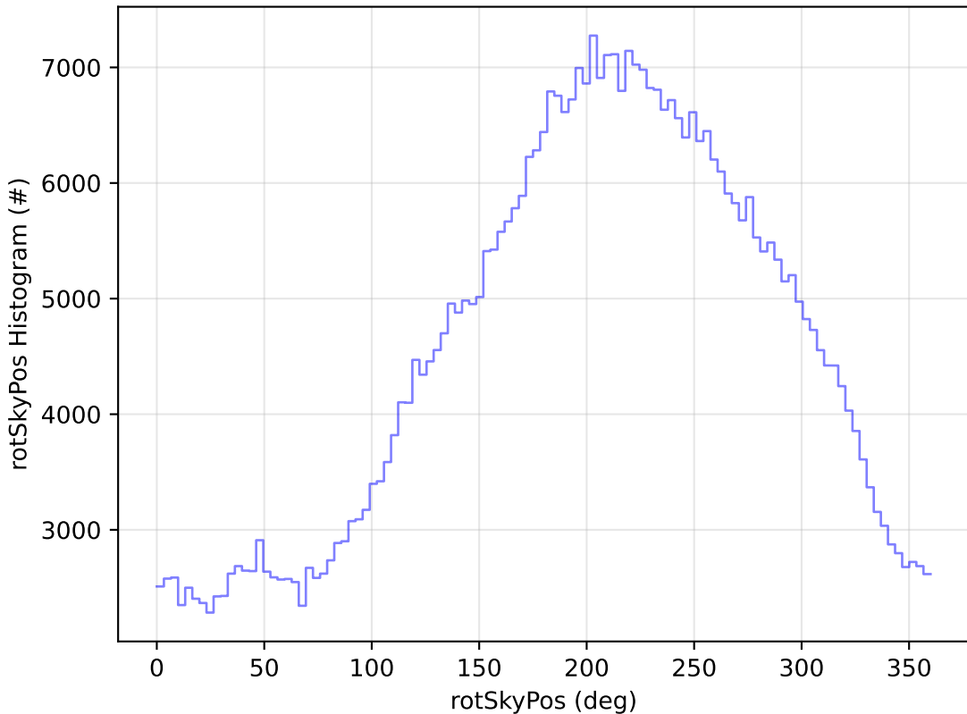
too_elab_r256_d2_ugrizy_v3.4_10yrs WFD i band: rotSkyPos Histogram
