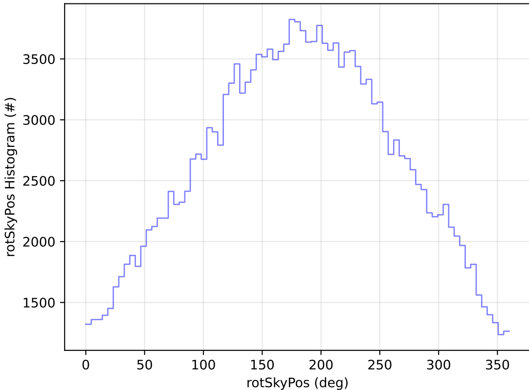
too_elab_r256_d2_ugrizy_v3.4_10yrs WFD g band: rotSkyPos Histogram
