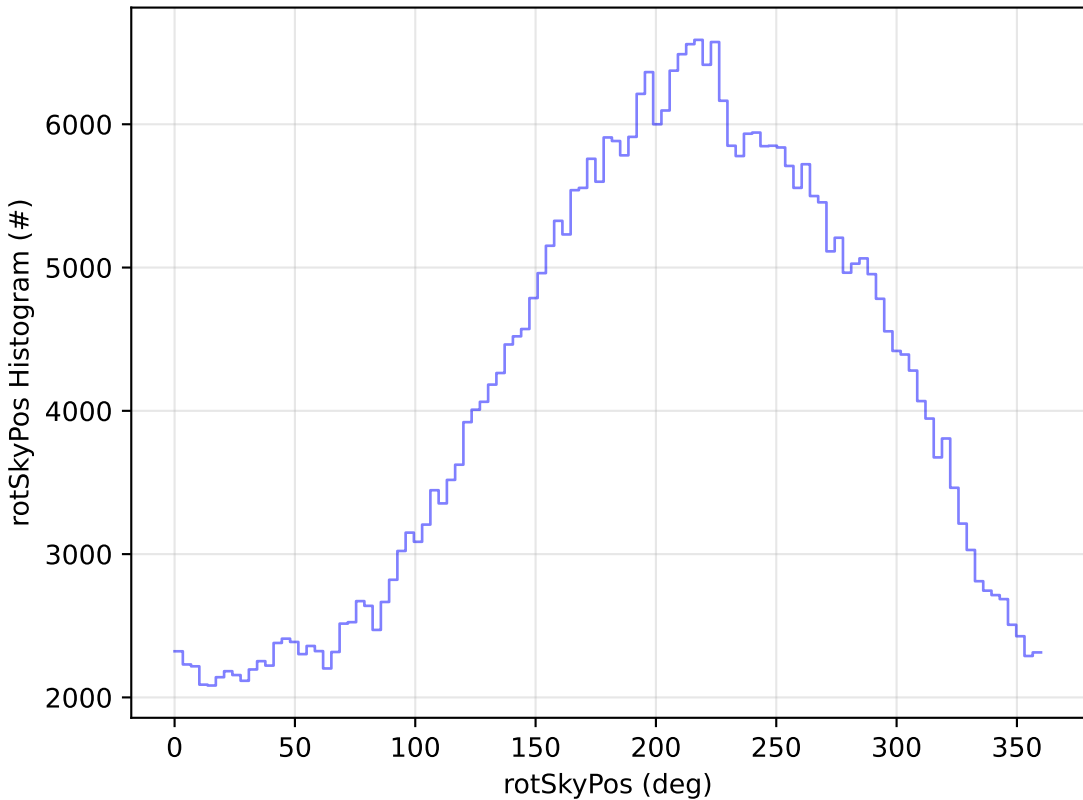
too_elab_r256_d2_ugrizy_v3.4_10yrs All sky z band: rotSkyPos Histogram
