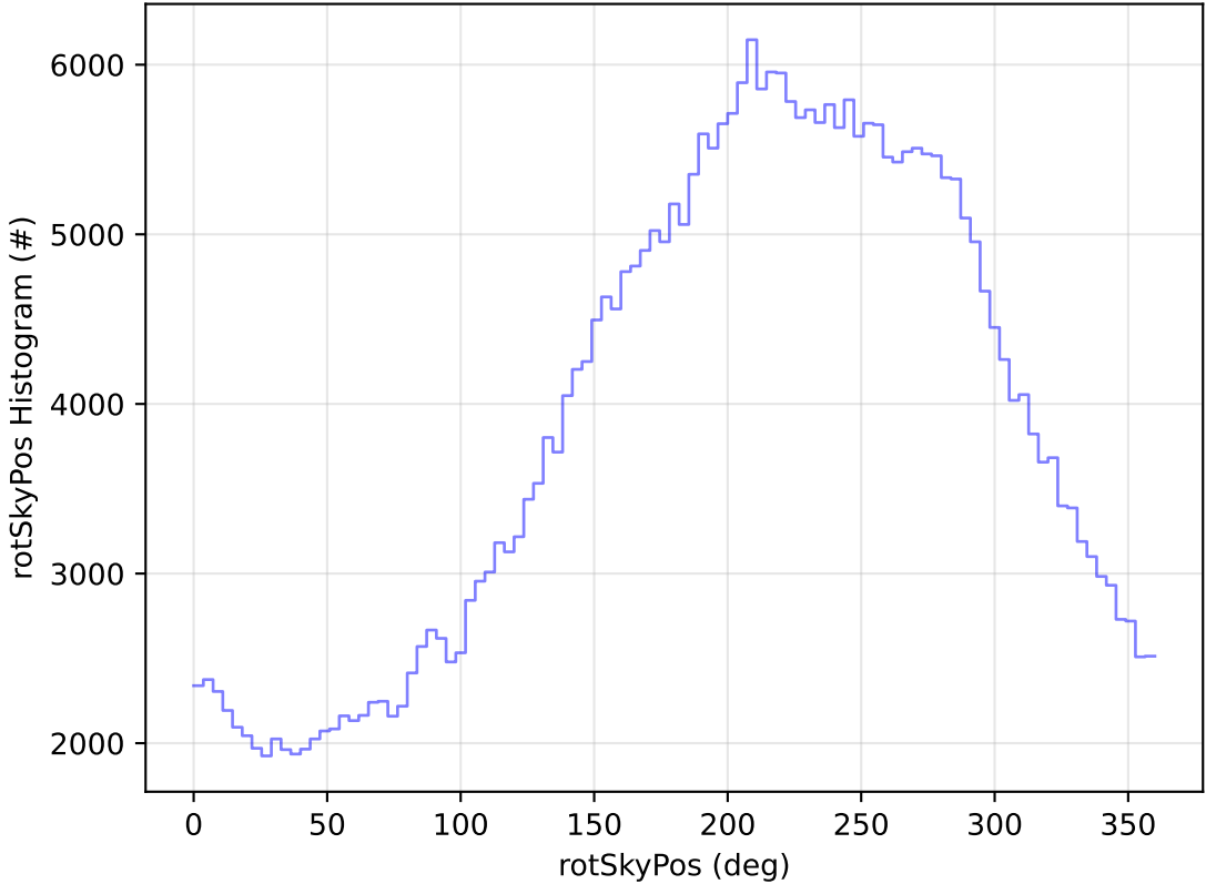
too_elab_r256_d2_ugrizy_v3.4_10yrs All sky y band: rotSkyPos Histogram
