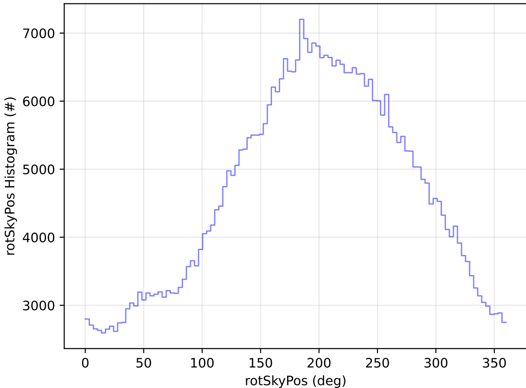
too_elab_r256_d2_ugrizy_v3.4_10yrs All sky r band: rotSkyPos Histogram
