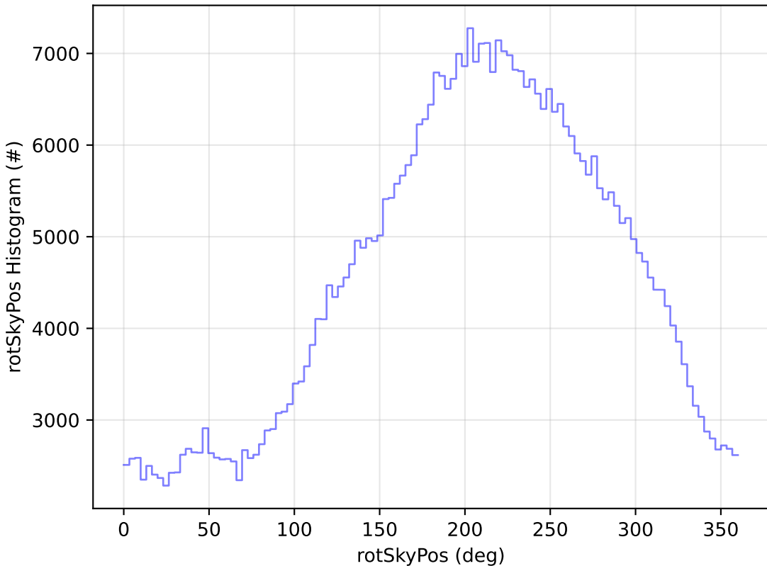
too_elab_r256_d2_ugrizy_v3.4_10yrs All sky i band: rotSkyPos Histogram
