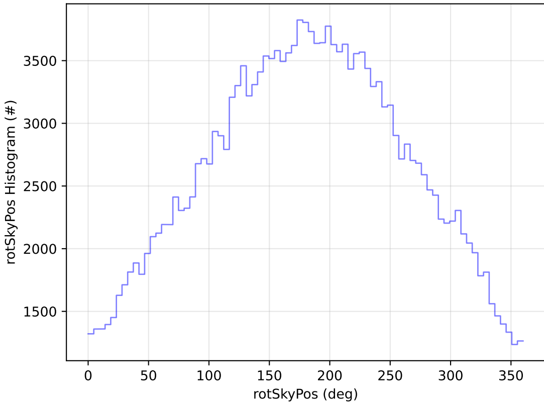
too_elab_r256_d2_ugrizy_v3.4_10yrs All sky g band: rotSkyPos Histogram
