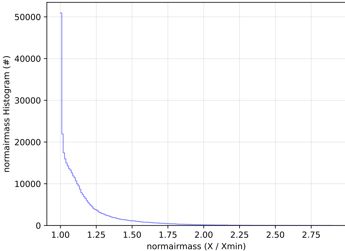
too_elab_r256_d2_ugrizy_v3.4_10yrs WFD y band: normairmass Histogram
