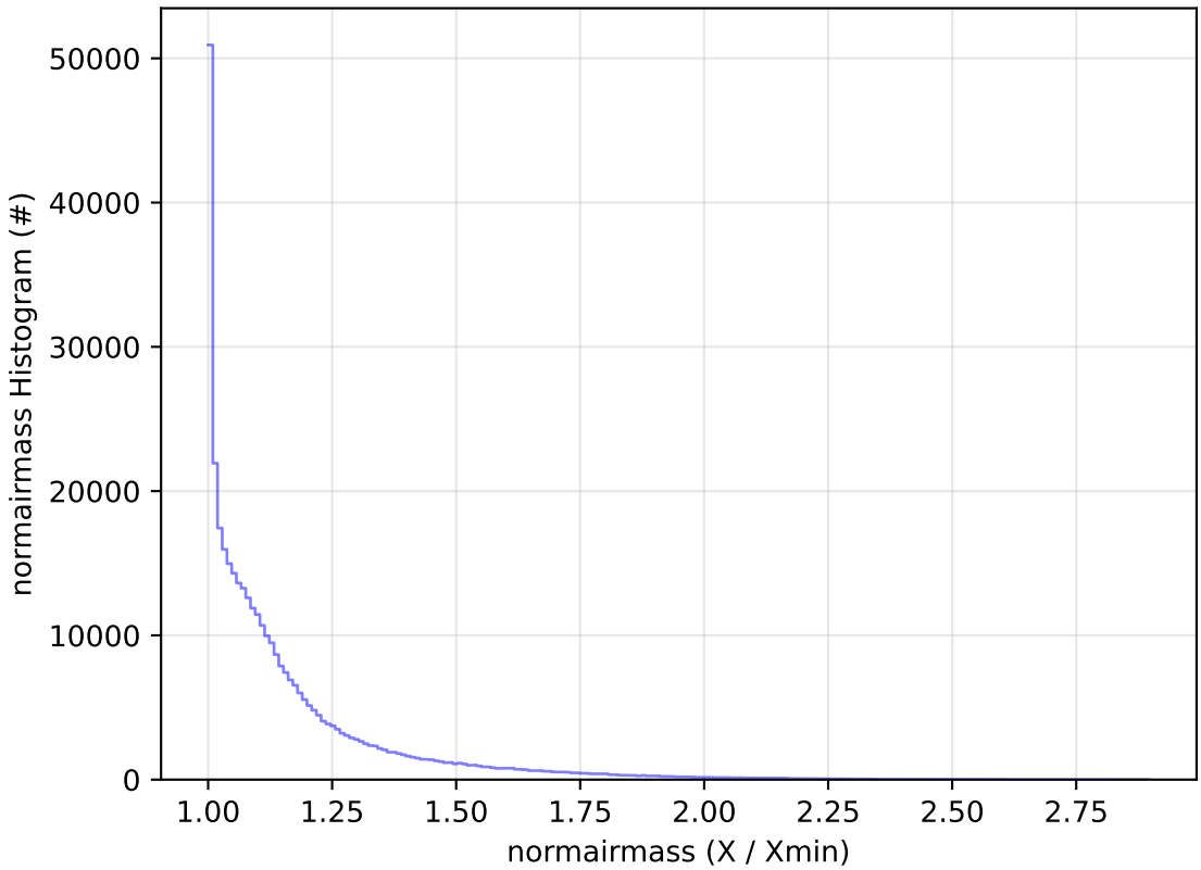
too_elab_r256_d2_ugrizy_v3.4_10yrs All sky y band: normairmass Histogram
