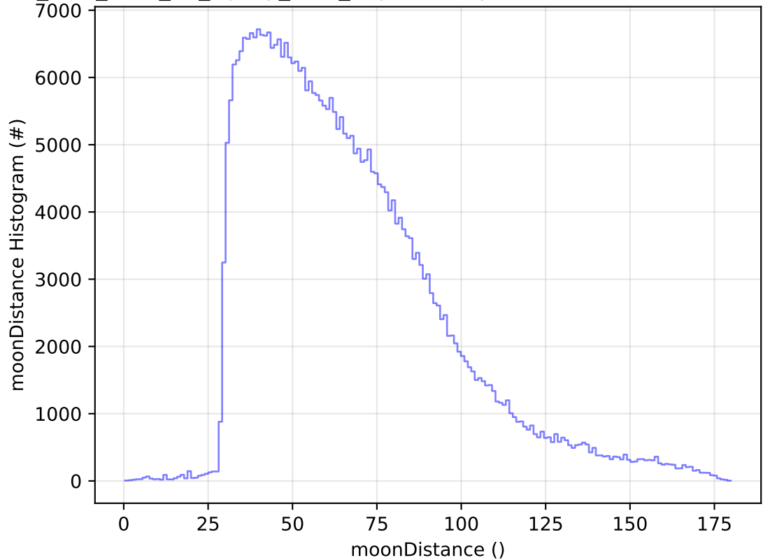
too_elab_r256_d2_ugrizy_v3.4_10yrs WFD y band: moonDistance Histogram
