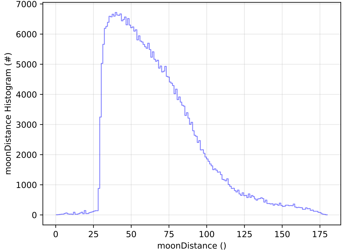
too_elab_r256_d2_ugrizy_v3.4_10yrs All sky y band: moonDistance Histogram
