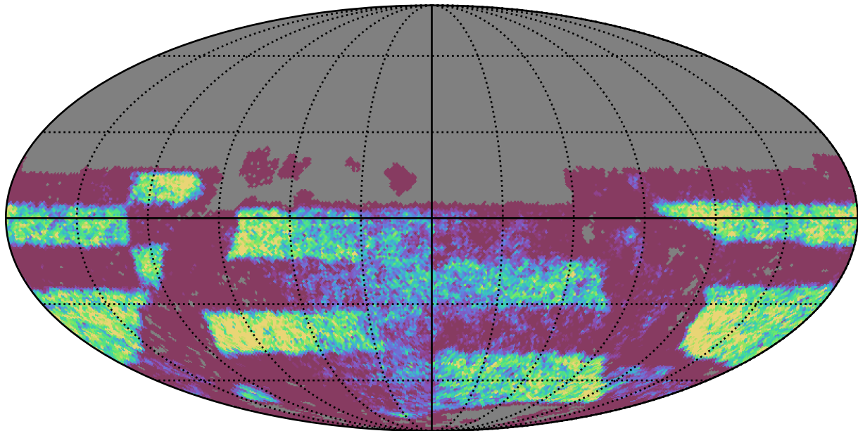
too_elab_r256_d2_ugrizy_v3.4_10yrs Yr 3-4 y band: NVisits
