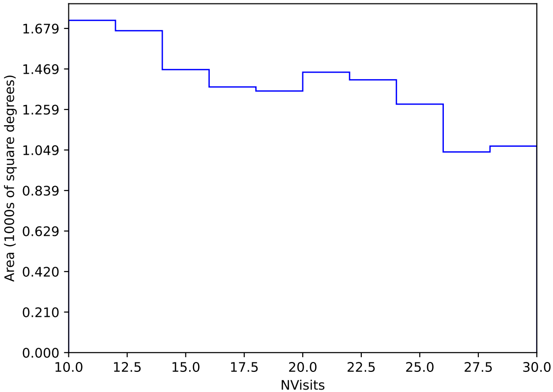
too_elab_r256_d2_ugrizy_v3.4_10yrs Yr 3-4 y band: NVisits
