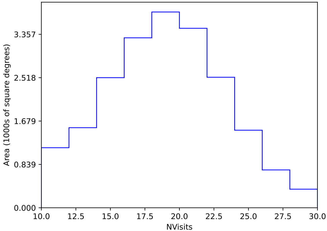
too_elab_r256_d2_ugrizy_v3.4_10yrs Yr 1 y band: NVisits
