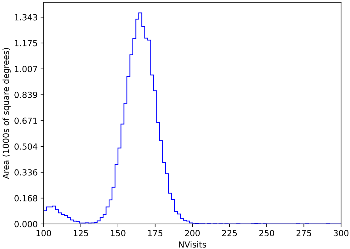
too_elab_r256_d2_ugrizy_v3.4_10yrs WFD y band: NVisits
