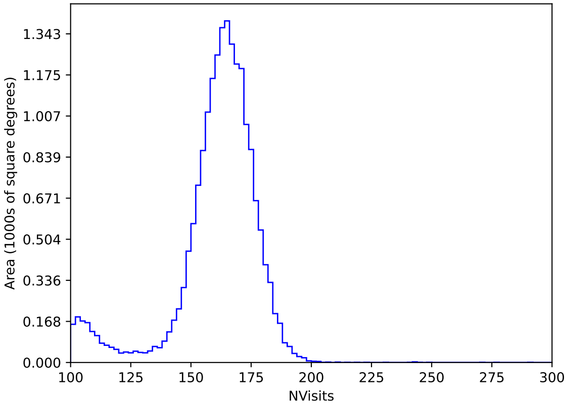
too_elab_r256_d2_ugrizy_v3.4_10yrs All sky y band: NVisits
