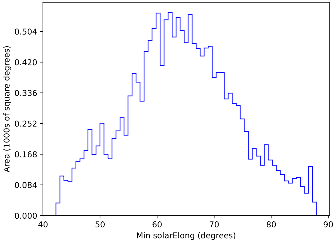
too_elab_r256_d2_ugrizy_v3.4_10yrs WFD y band: Min solarElong
