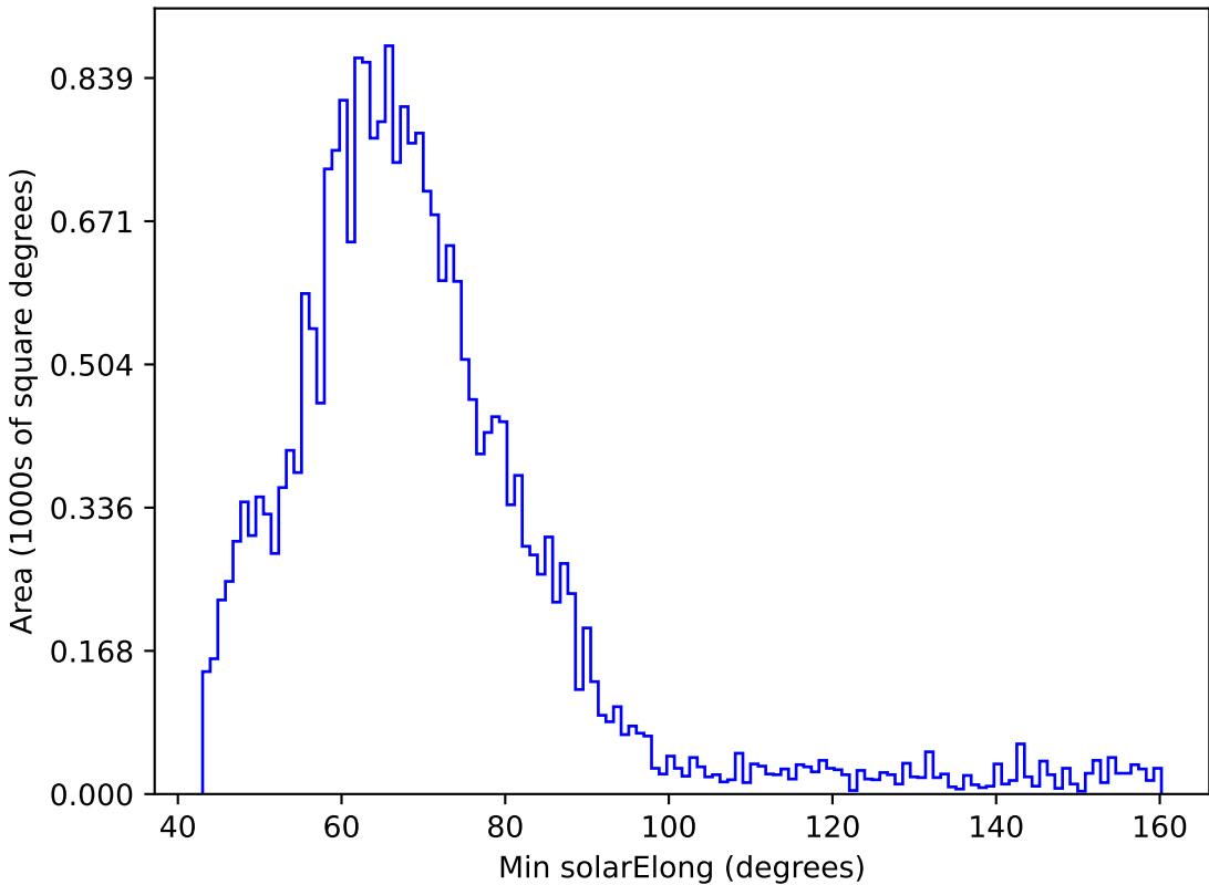
too_elab_r256_d2_ugrizy_v3.4_10yrs All sky y band: Min solarElong
