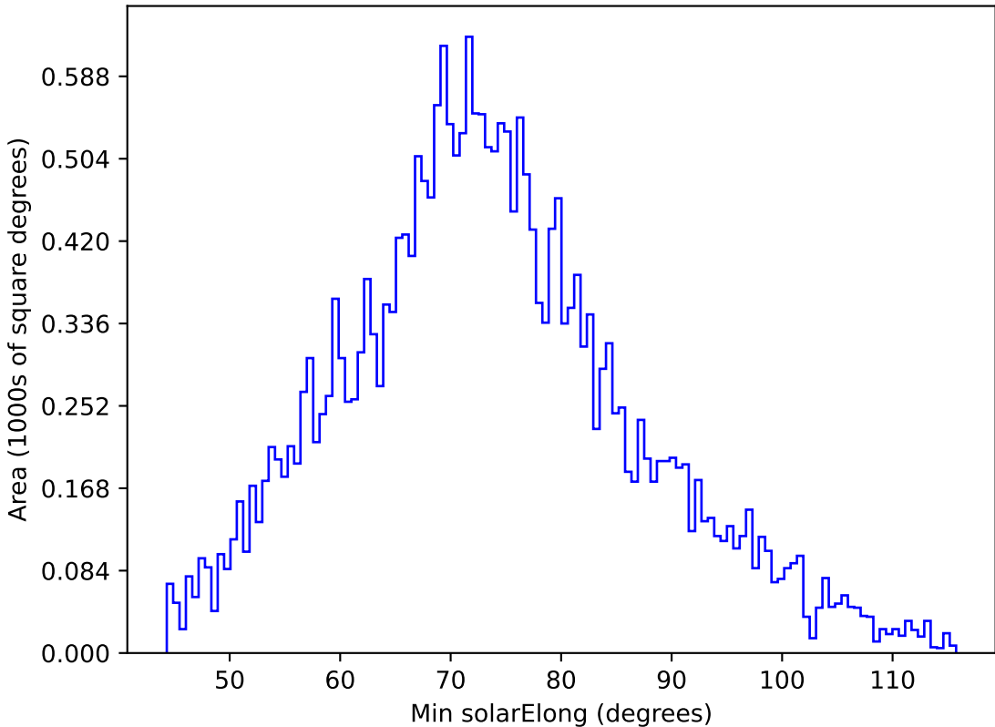
too_elab_r256_d2_ugrizy_v3.4_10yrs All sky g band: Min solarElong
