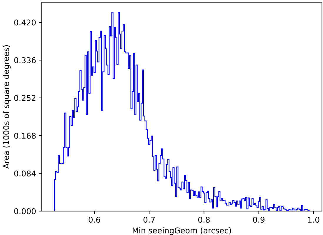
too_elab_r256_d2_ugrizy_v3.4_10yrs Yr 1 y band: Min seeingGeom
