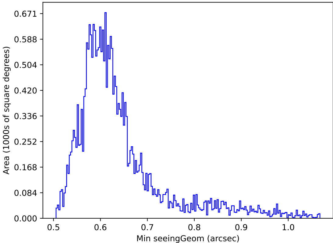
too_elab_r256_d2_ugrizy_v3.4_10yrs Yr 1 i band: Min seeingGeom
