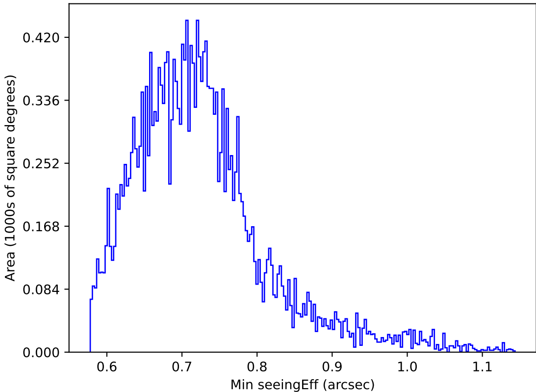
too_elab_r256_d2_ugrizy_v3.4_10yrs Yr 1 y band: Min seeingEff
