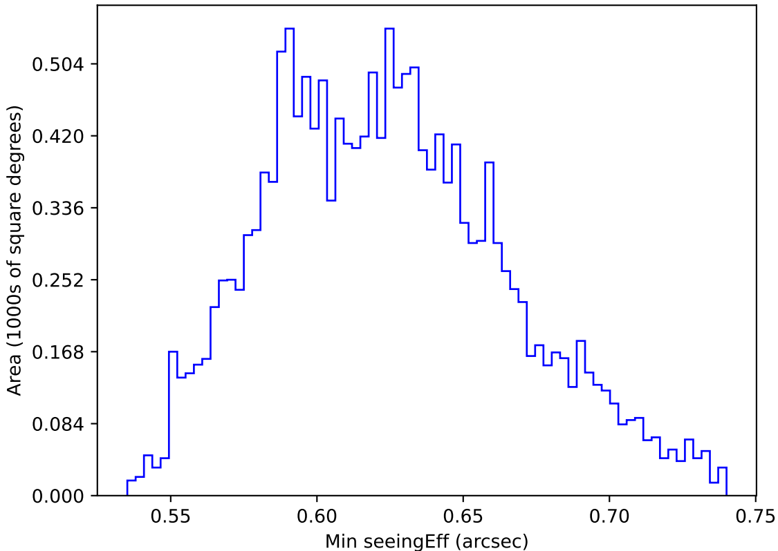
too_elab_r256_d2_ugrizy_v3.4_10yrs WFD y band: Min seeingEff
