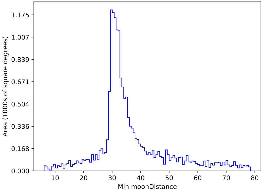
too_elab_r256_d2_ugrizy_v3.4_10yrs WFD r band: Min moonDistance
