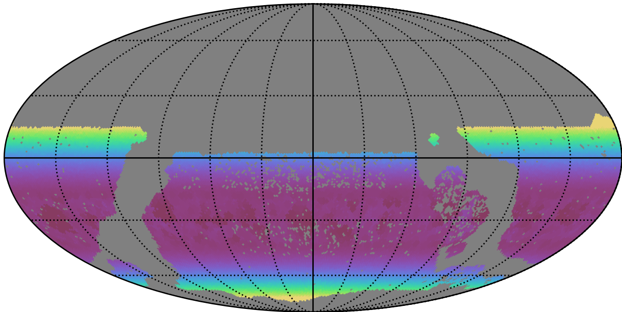
too_elab_r256_d2_ugrizy_v3.4_10yrs WFD y band: Min airmass
