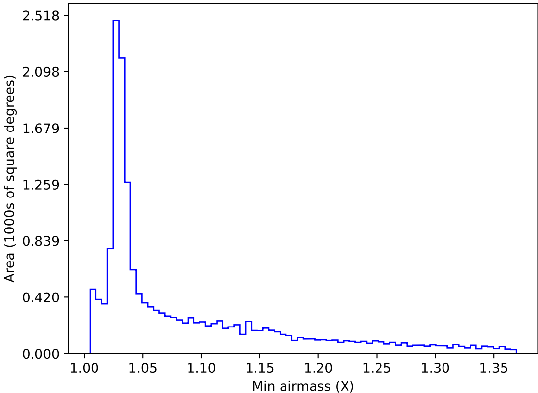
too_elab_r256_d2_ugrizy_v3.4_10yrs WFD y band: Min airmass
