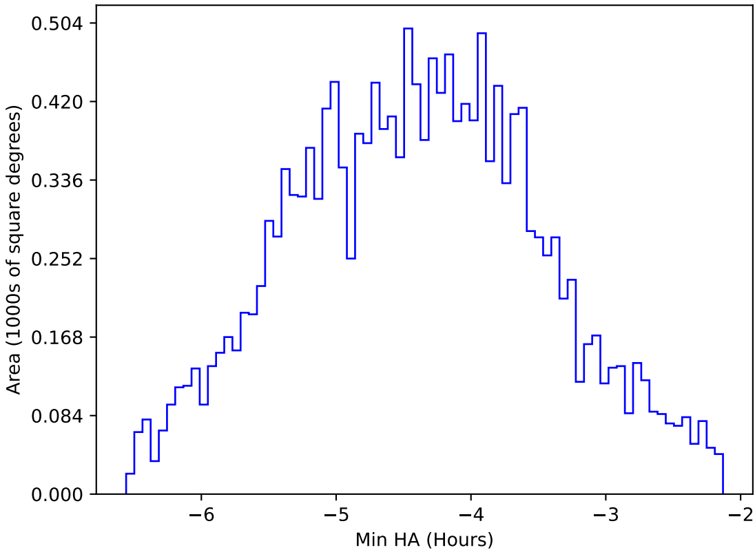
too_elab_r256_d2_ugrizy_v3.4_10yrs WFD z band: Min HA
