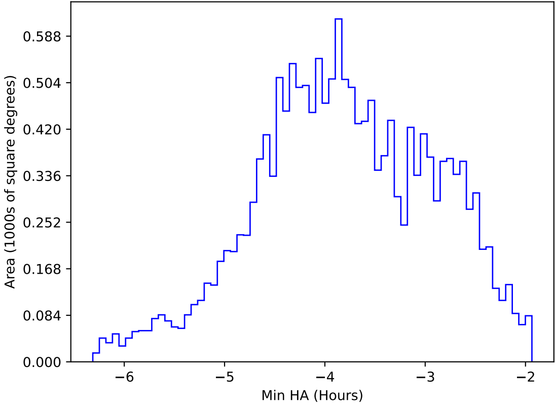
too_elab_r256_d2_ugrizy_v3.4_10yrs WFD y band: Min HA
