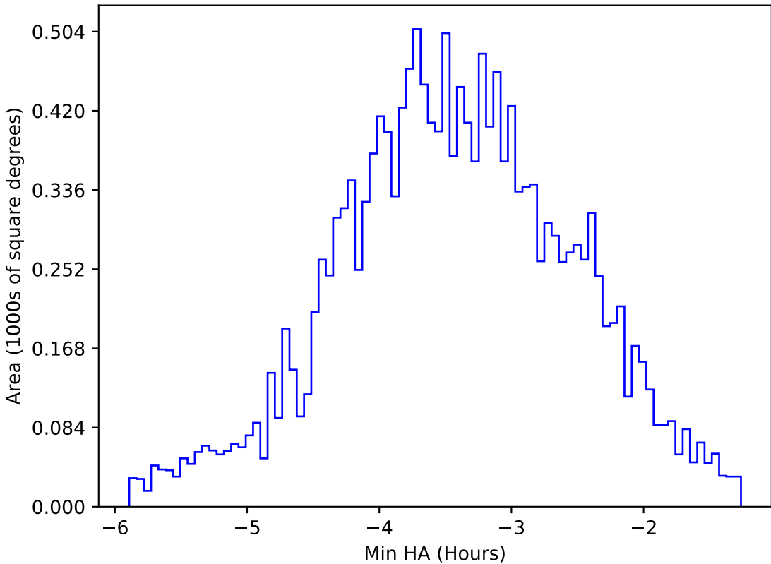
too_elab_r256_d2_ugrizy_v3.4_10yrs WFD u band: Min HA
