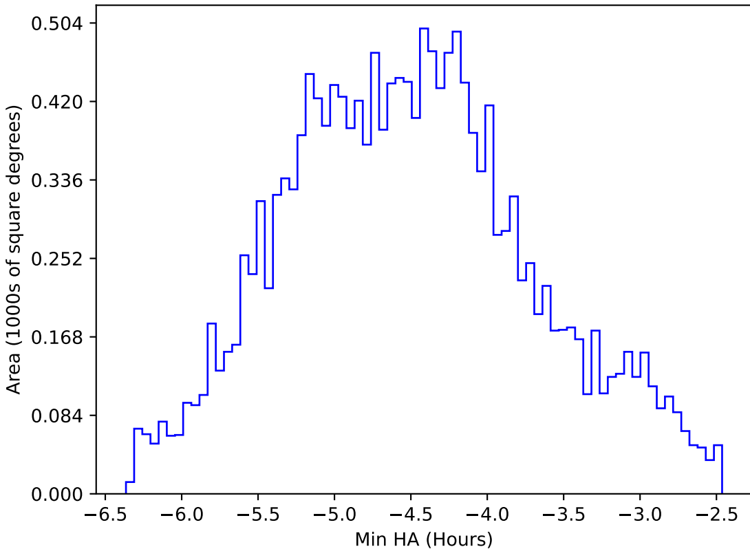
too_elab_r256_d2_ugrizy_v3.4_10yrs WFD r band: Min HA
