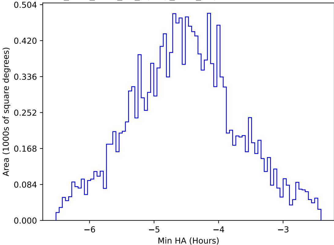
too_elab_r256_d2_ugrizy_v3.4_10yrs WFD i band: Min HA
