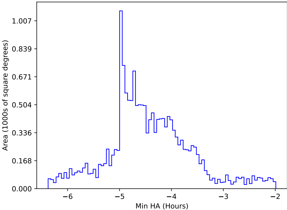
too_elab_r256_d2_ugrizy_v3.4_10yrs WFD g band: Min HA
