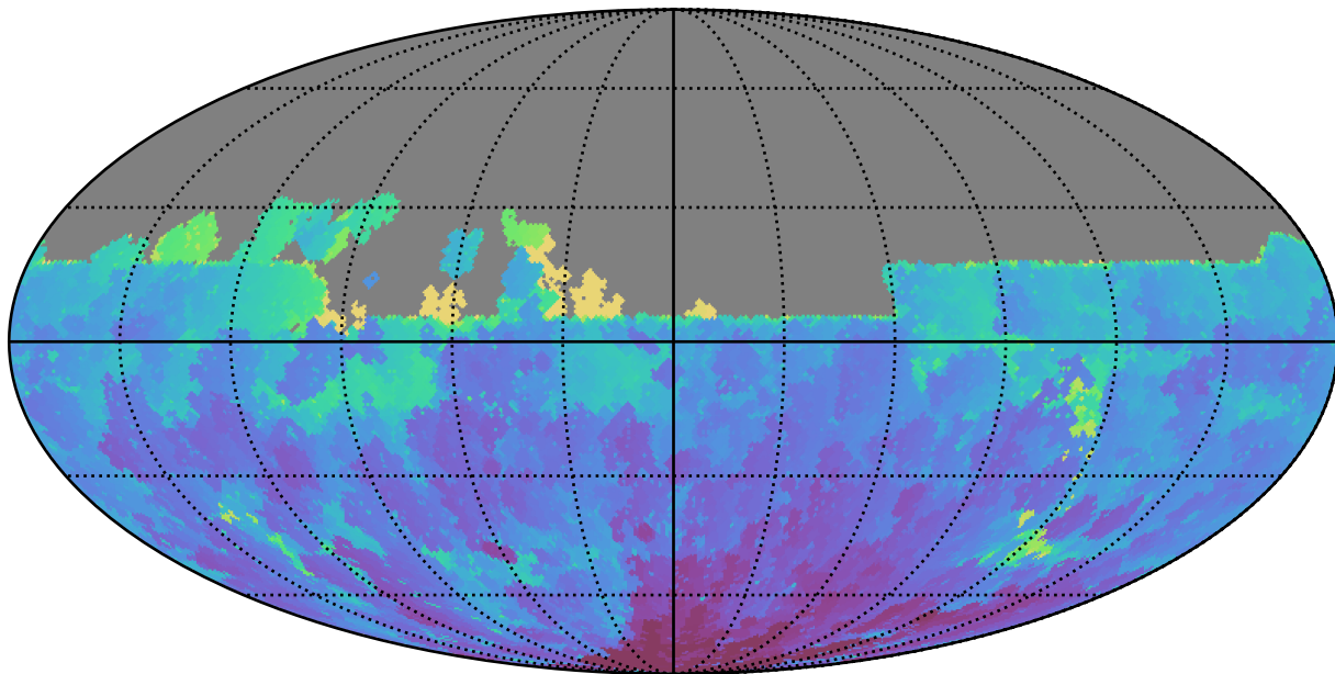
too_elab_r256_d2_ugrizy_v3.4_10yrs All sky u band: Min HA
