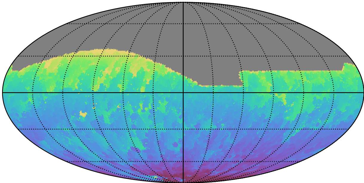
too_elab_r256_d2_ugrizy_v3.4_10yrs All sky i band: Min HA
