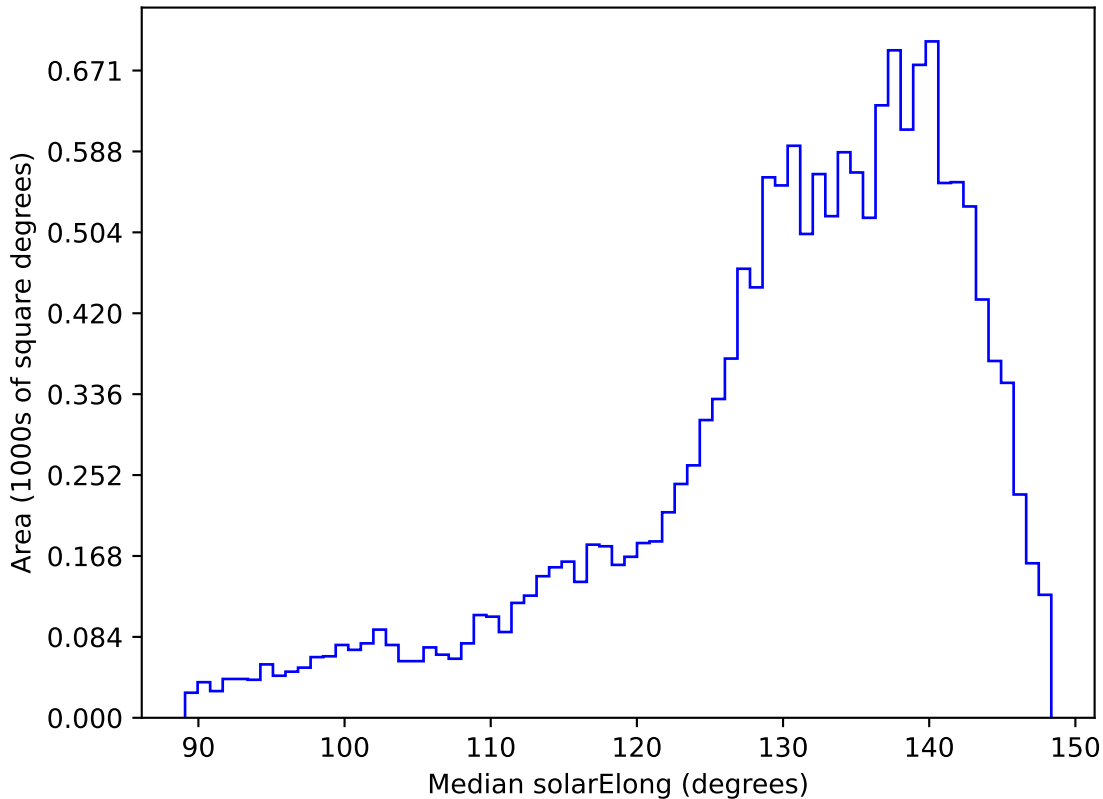
too_elab_r256_d2_ugrizy_v3.4_10yrs WFD y band: Median solarElong
