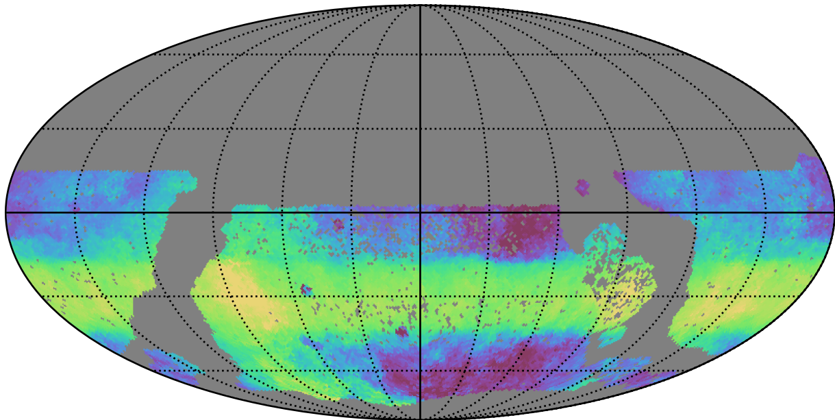
too_elab_r256_d2_ugrizy_v3.4_10yrs WFD y band: Median HA
