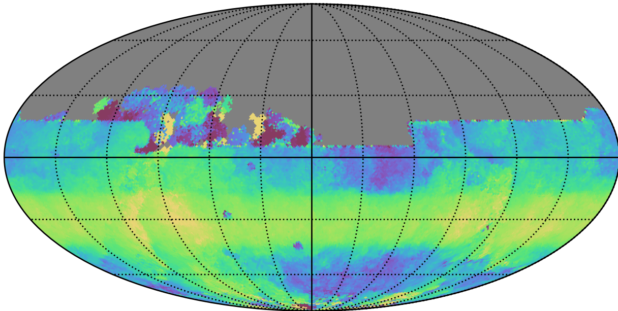
too_elab_r256_d2_ugrizy_v3.4_10yrs All sky y band: Median HA
