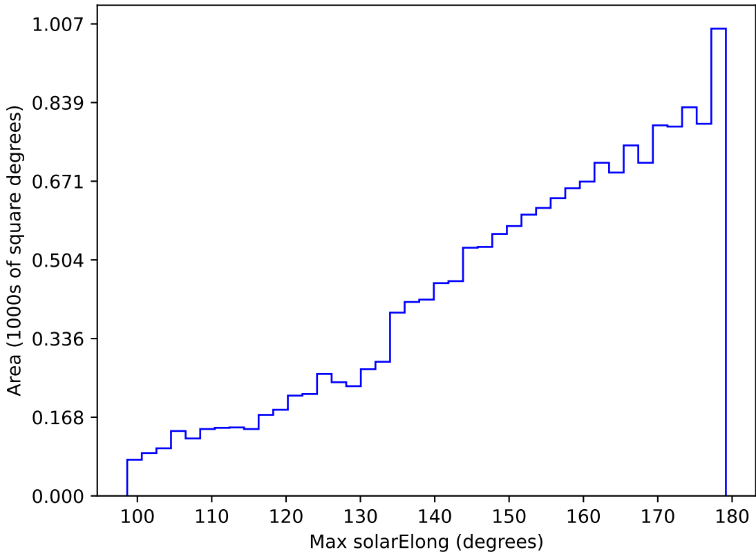
too_elab_r256_d2_ugrizy_v3.4_10yrs WFD y band: Max solarElong
