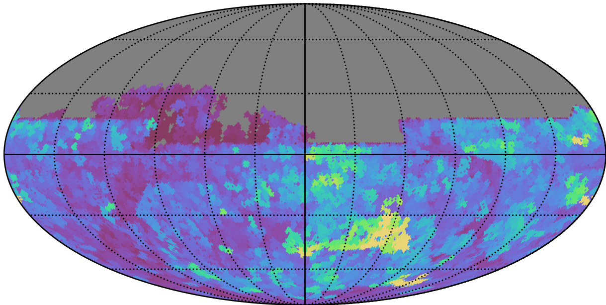
too_elab_r256_d2_ugrizy_v3.4_10yrs All sky y band: Max seeingEff
