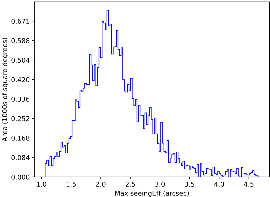
too_elab_r256_d2_ugrizy_v3.4_10yrs All sky y band: Max seeingEff
