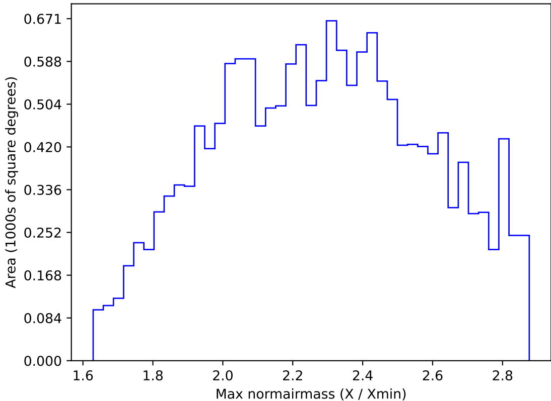
too_elab_r256_d2_ugrizy_v3.4_10yrs WFD z band: Max normairmass
