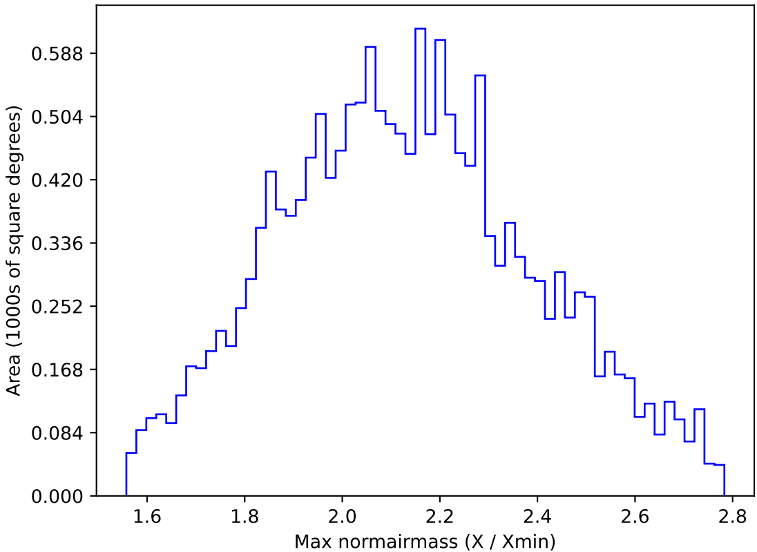
too_elab_r256_d2_ugrizy_v3.4_10yrs WFD y band: Max normairmass
