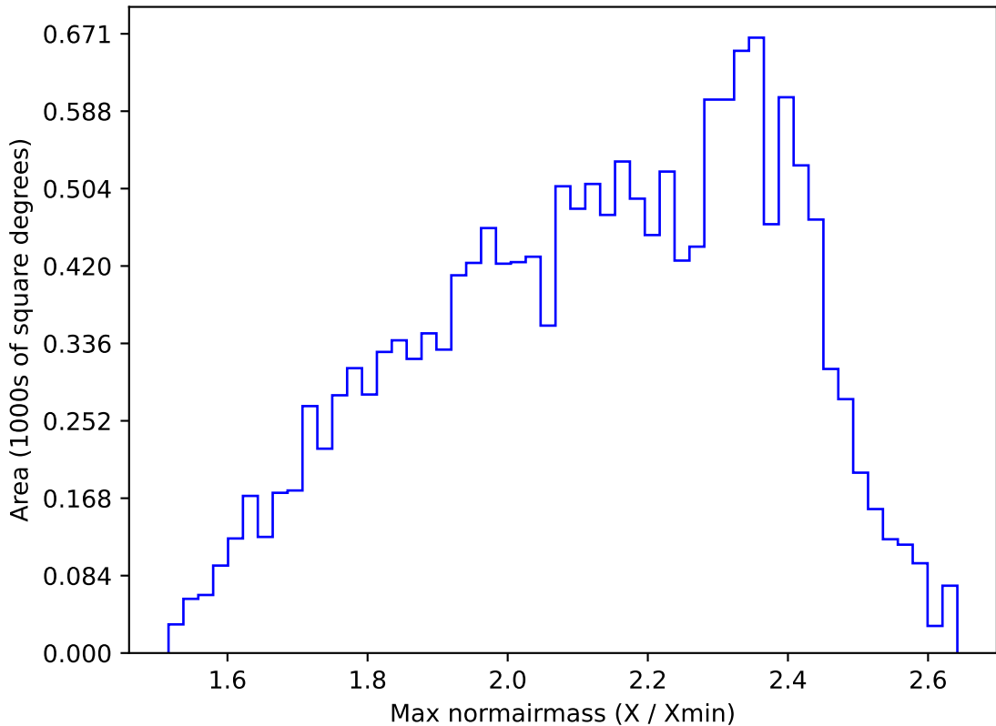
too_elab_r256_d2_ugrizy_v3.4_10yrs WFD r band: Max normairmass
