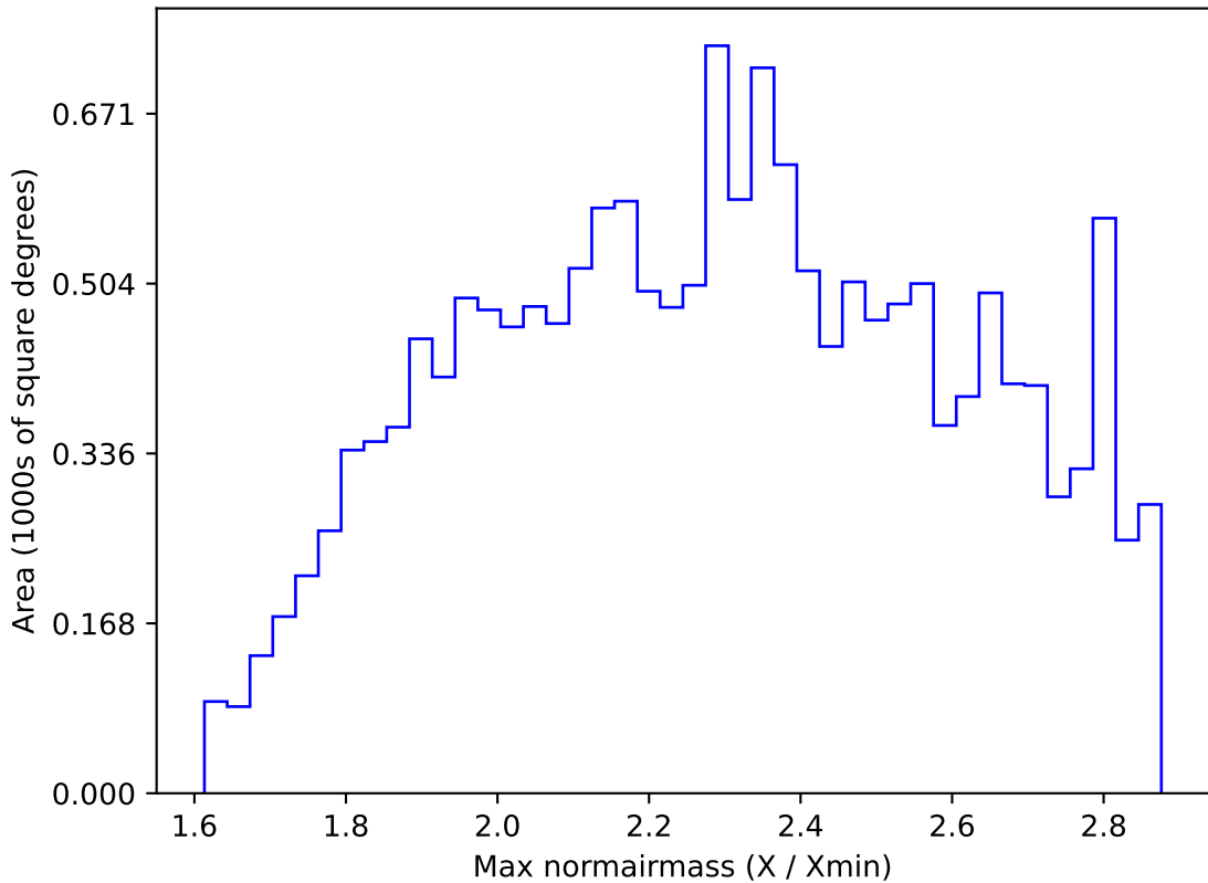
too_elab_r256_d2_ugrizy_v3.4_10yrs WFD i band: Max normairmass
