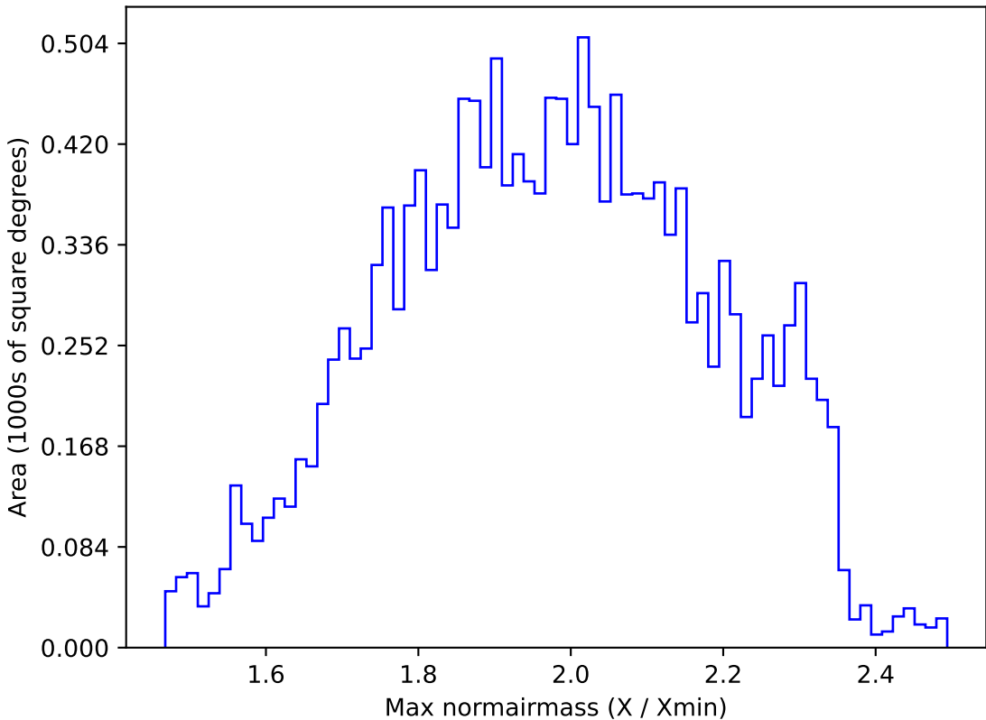
too_elab_r256_d2_ugrizy_v3.4_10yrs WFD g band: Max normairmass
