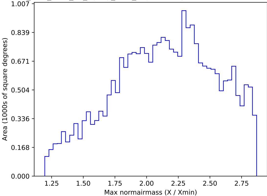
too_elab_r256_d2_ugrizy_v3.4_10yrs All sky i band: Max normairmass
